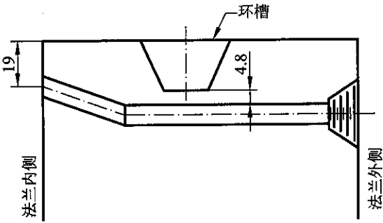
图 A.7.3 环连接面法兰用测压孔结构
