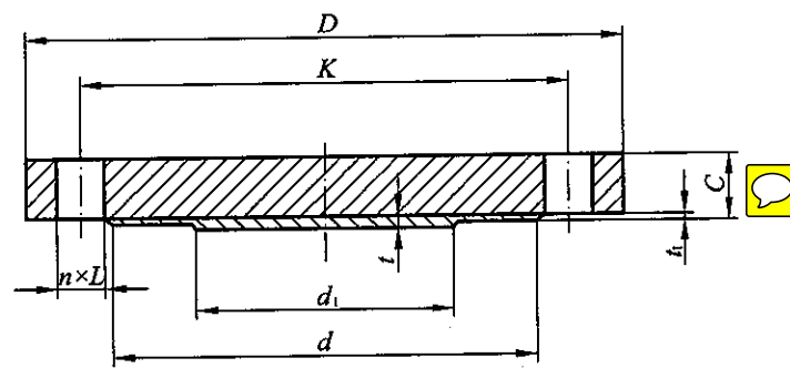
突面 (RF)
