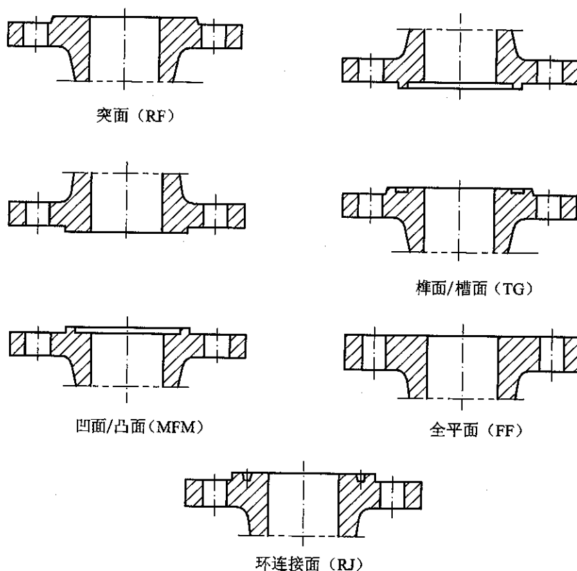
图 3.2.1 密封面型式
