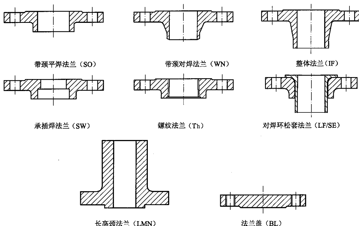
图 3.1.1 法兰类型
