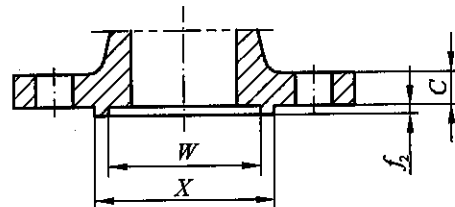
榫面 (T)
