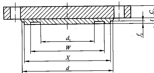
榫面 (T)
