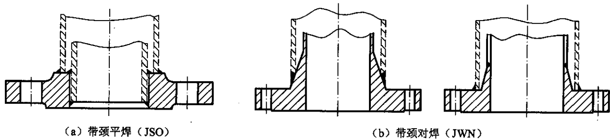
图 B.3.1 夹套法兰类型 表 B.3.1 法兰类型代号
