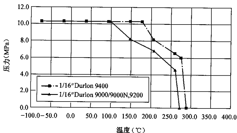
图 A.0.4-2 填充改性聚四氟乙烯垫片压力-温度图
