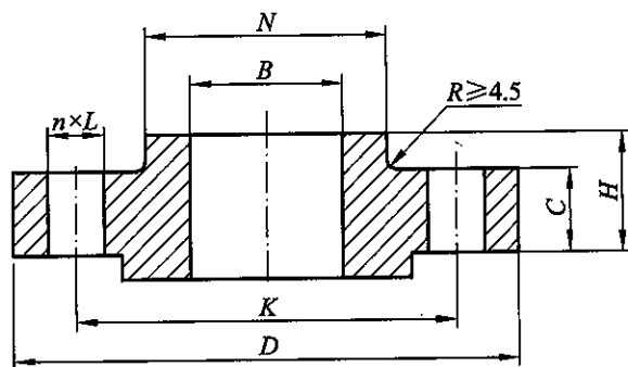
图 B.6.2-1 带颈平焊夹套法兰
