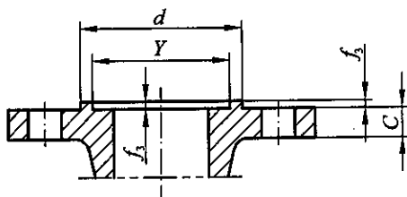
凹面 (FM)
