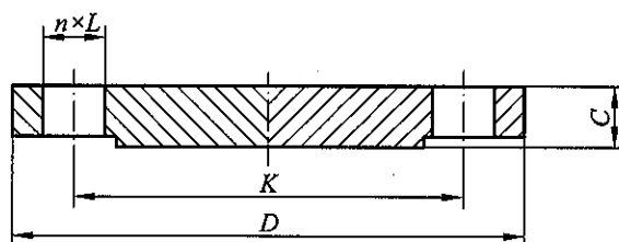
图 8.2.9 钢制管法兰
