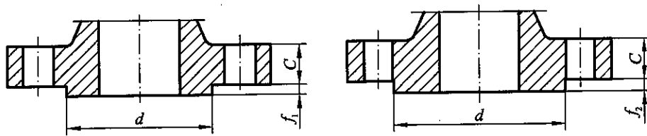
图 3.2.5-1 突面(RF)法兰的密封面尺寸
