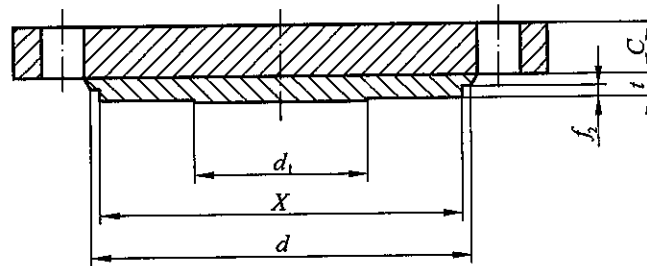
凸面 (M)
