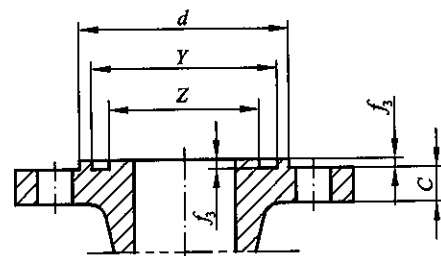
槽面 (G)
